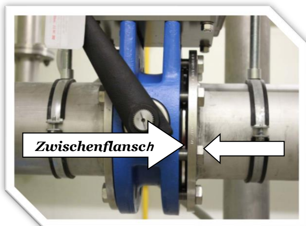
Kaum erkennbar: Seitenansicht des eingebauten AS54 Ventils
